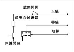
接線圖原理
