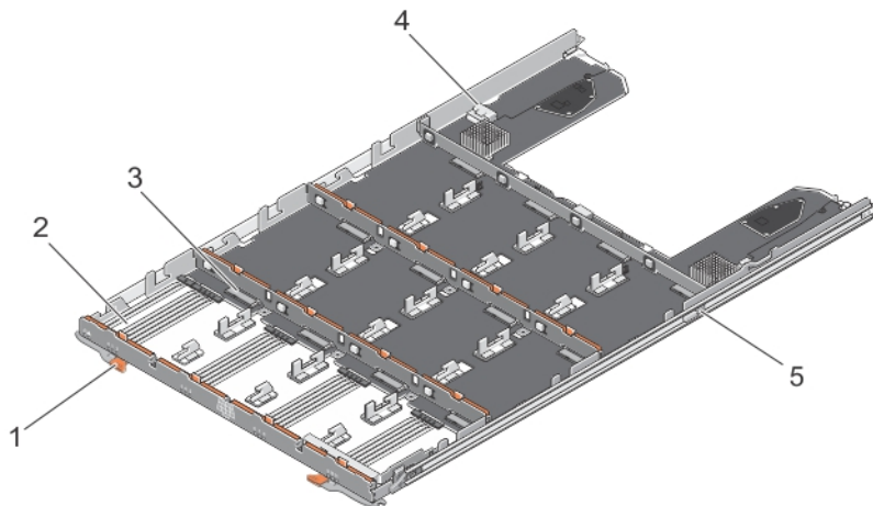
図 16. 物理ディスクドロワーの内部
