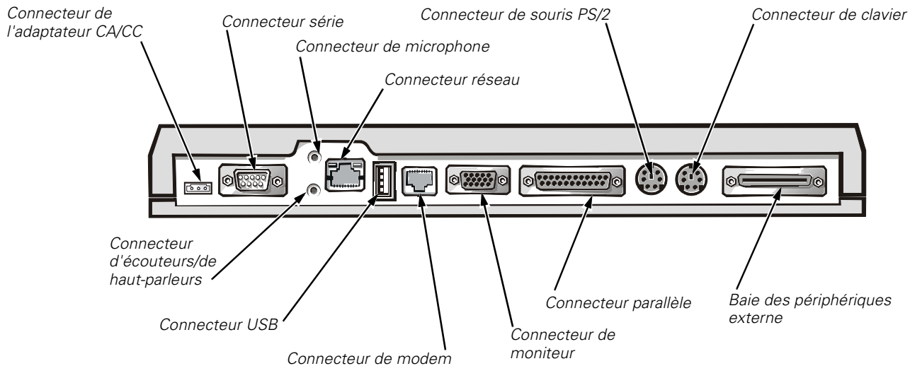
Figure 6-1. Connexion de périphériques externes à l'APR
