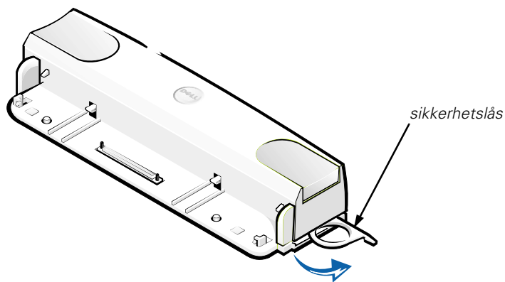
Figur 10-4. Sikkerhetslås for portreplikator
