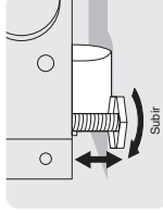
Rueda fija delantera con tornillo nivelador (algunos modelos)
